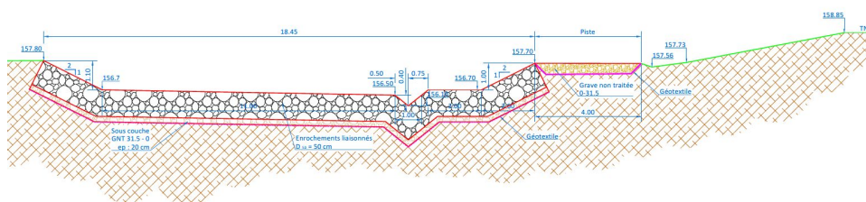
Coupe du Seuil Coupe BB
